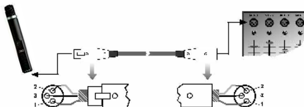
Figure 3: Branchement à l'aide d'un câble symétrique XLR
