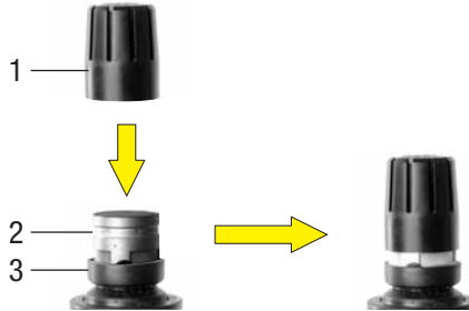
Abbildung 6: PPC1000/PB1000 montieren
