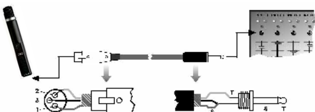
Figura 4: Conexão por meio de cabo não balanceado
