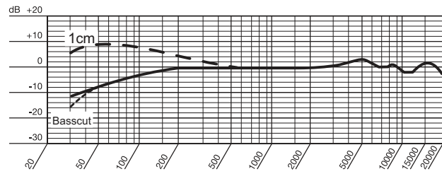
Risposta in frequenza (ipercardioid)
