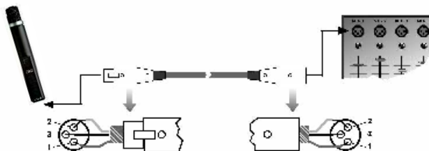
Figure 5: Branchement à l'aide d'un câble symétrique XLR
