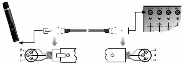
Abbildung 3: Anschluss über symmetrisches XLR-Kabel
