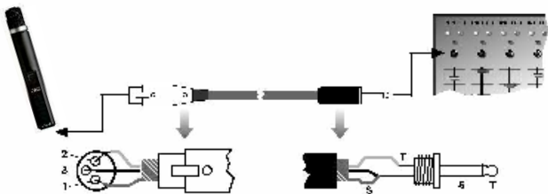
Abbildung 4: Anschluss über asymmetrisches Kabel
