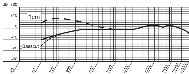
Risposta in frequenza (cardioide)
