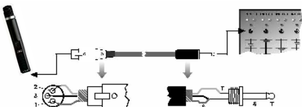
Figura 4: Conexión con cable no balanceado
