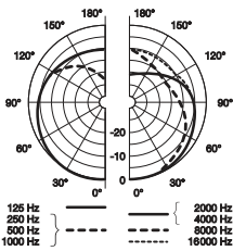
Diagramma polare (ipercardioid)
