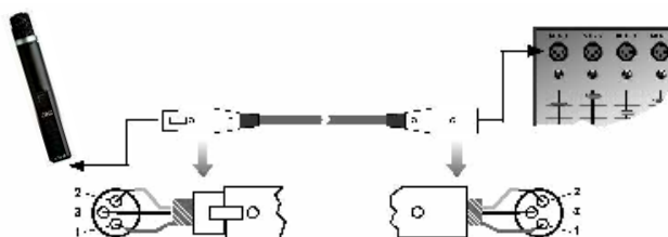
Figura 3: Conexión con cable XLR balanceado
