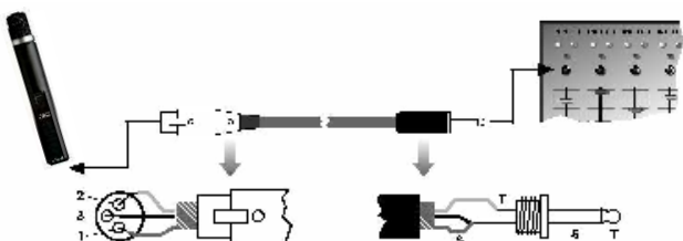
Figure 4: Branchement à l'aide d'un câble asymétrique
