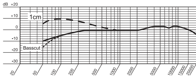
Resposta de frequência (cardióide)
