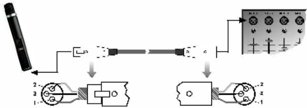
Abbildung 5: Anschluss über symmetrisches XLR-Kabel
