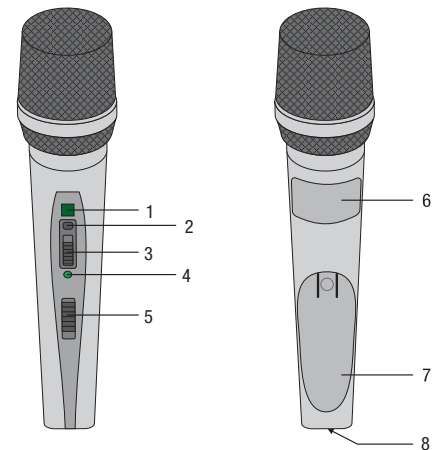
Abbildung 3: Bedienelemente des Senders HT420
