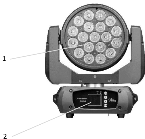
VISTA FRONTALE
