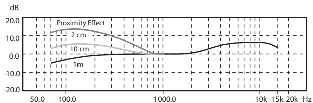
Grafico della risposta frequenza
