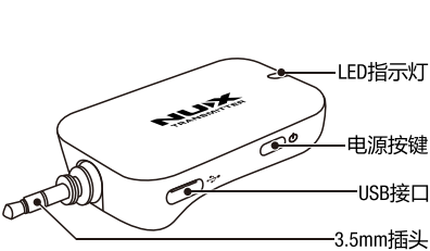
发射器
