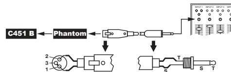
Abbildung 2: Anschluss an unsymmetrischen Eingang
