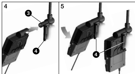
Fig. 3: Fixar o adaptador com o emissor de bolso no cone de microfone
