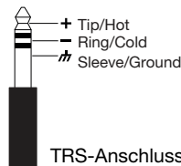
TRS-Anschluss
